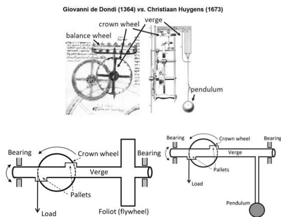
Рис. 7. Сравнение биянцевых часов Джованни де Донди (1364 г., Падуа) из его Tractatus Astrarii , и вторых маятниковых часов, построенных Кристианом Гюйгенсом (1673 г.); рисунок из его Horologium Oscillatorium и кинематические схемы обоих механизмов
